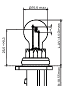
P13W
