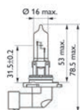
HB3
