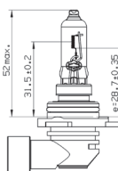
HIR2
