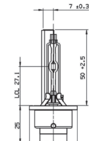
D2S
