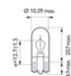
W2,2W-W2,5W W3W-W5W(Y)
