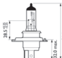
H4
